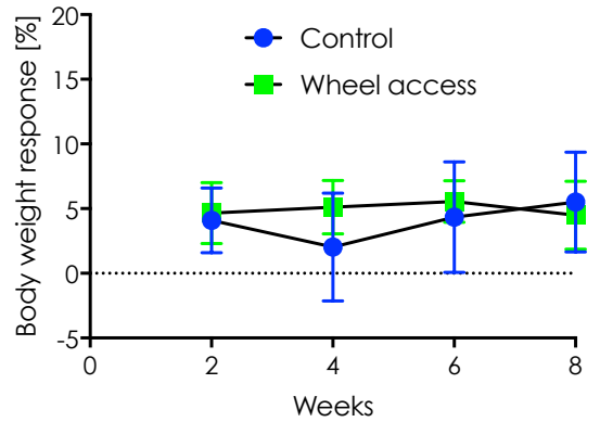
CC037/TauUnc
